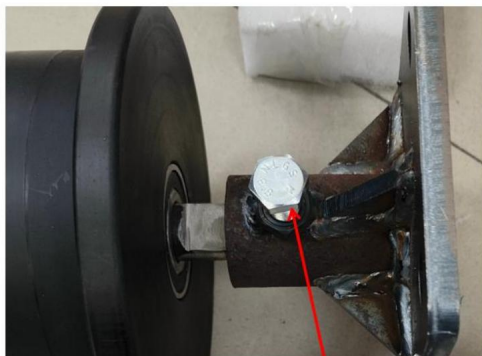
Bolt
