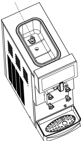
Niveau-Schwimmer
