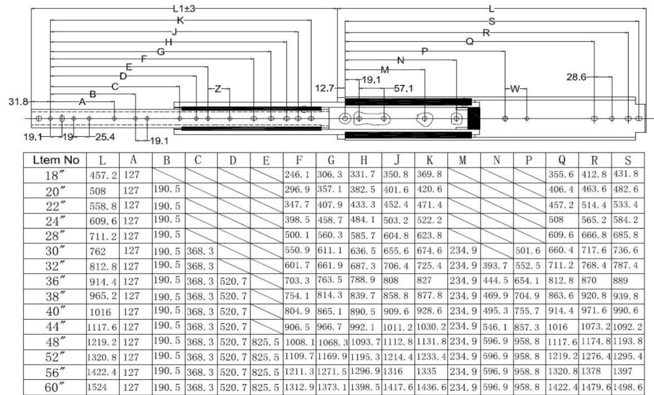
7601 Patrón de orificios de instalación (Unidades: mm:
