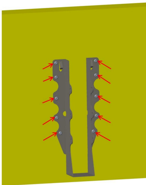
2.10 śrub mocujących wieszak belki nośnej do belki
