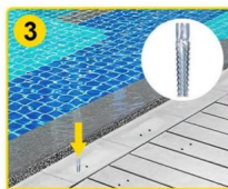
Insert Anchors
