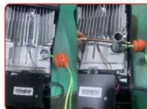
Fase 4 Aprire il coperchio del pulsante ed estrarre la candela di accensione con una chiave speciale
