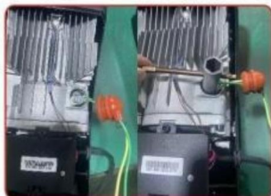
Passaggio 3 Il terzo passaggio consiste nell'aprire il tappo fibbia, rimuovere la candela di accensione con chiave speciale
