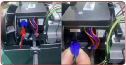
Paso 2 Desconecte el enchufe de encendido
