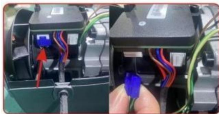
Étape 2 Débranchez la bougie d'allumage
