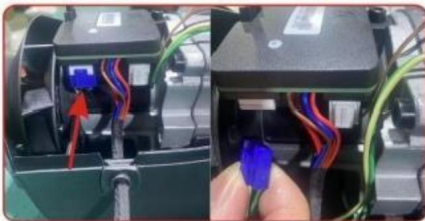
Fase 2 Scollegare la candela di accensione
