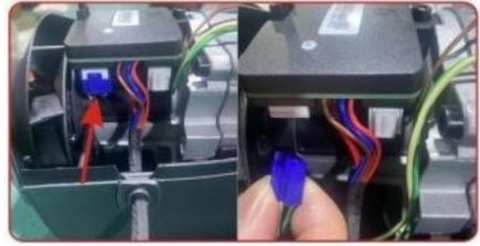
Stap 2: Trek de contactplug uit het contact
