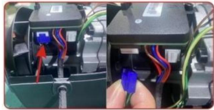
Steg 2 Koppla ur tändstiftet
