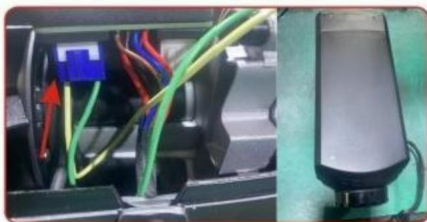
Krok 3 Trzecim krokiem jest otwarcie zaślepka, wyjmij świecę zapłonową ze specjalnym kluczem
