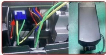
Paso 3 El tercer paso es abrir el tapa de hebilla, quitar bujía de encendido con llave especial
