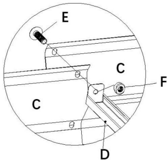
3. De verbinding van een drijfstaang met een rechte plaat.
