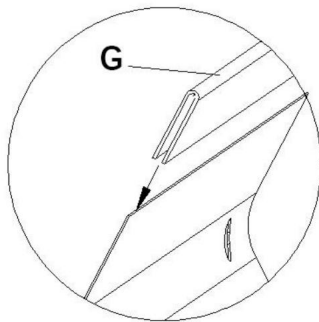
4. Installieren Sie den Gummiverkleidungsstreifen.
