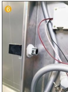
6 Sätt in handspraymunstycket i panelen och installera packningen.
