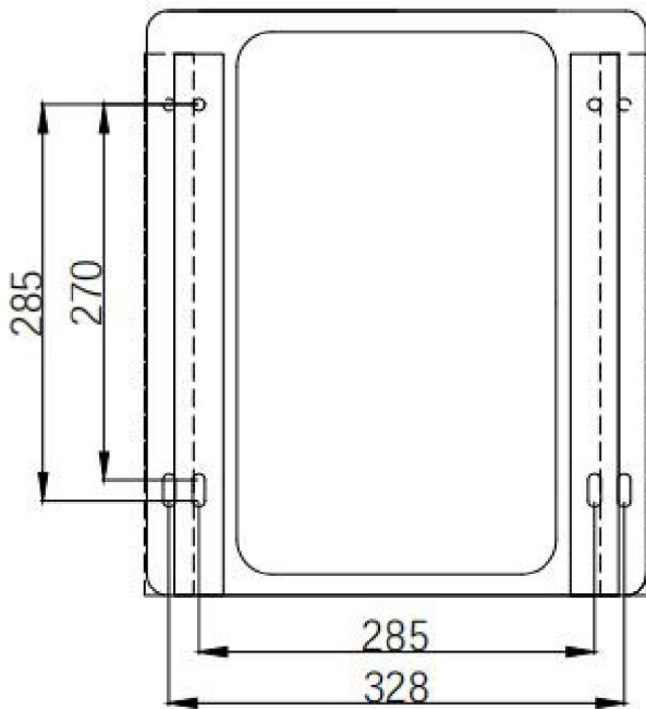
Dimensiones de montaje del asiento de la carretilla elevadora
