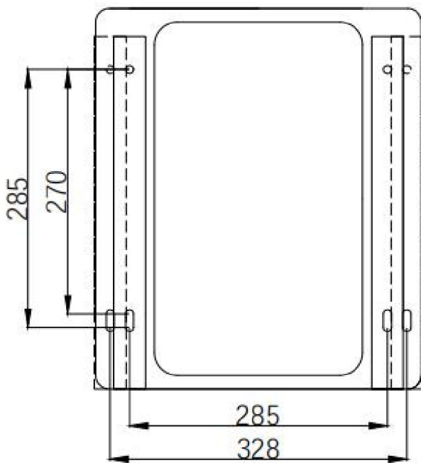
Dimensioni di montaggio del sedile del carrello elevatore
