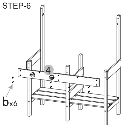
STEP-6
