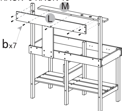
KROK -9 KROK-10
