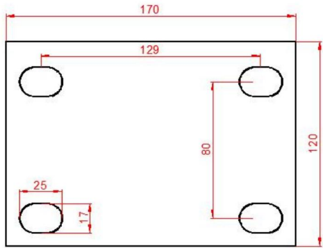
Parámetros de los orificios de montaje (mm)
