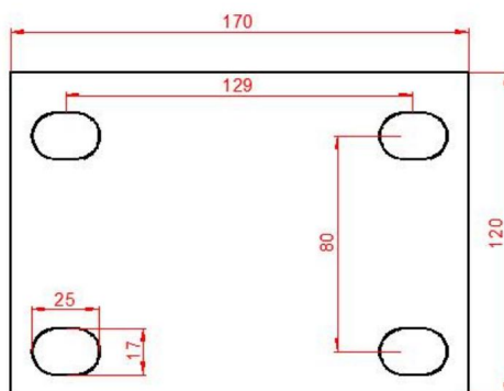
Paramètres des trous de montage (mm)
