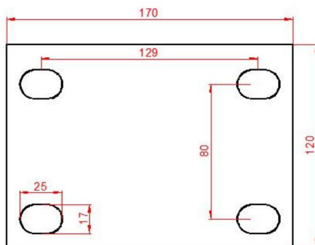
Parameters van montagegaten (mm)
