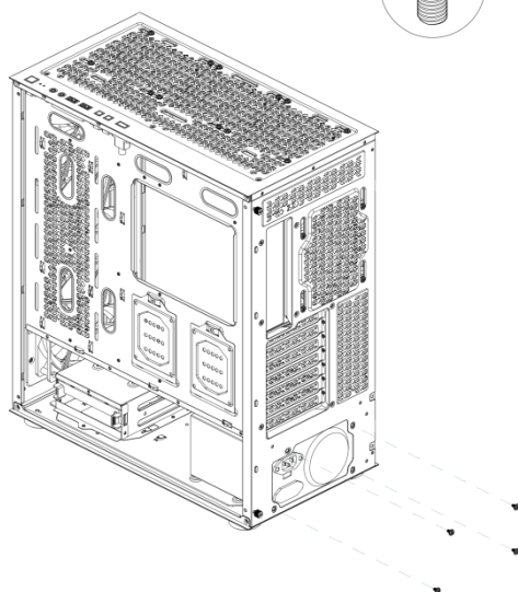
Installation de l'alimentation électrique
