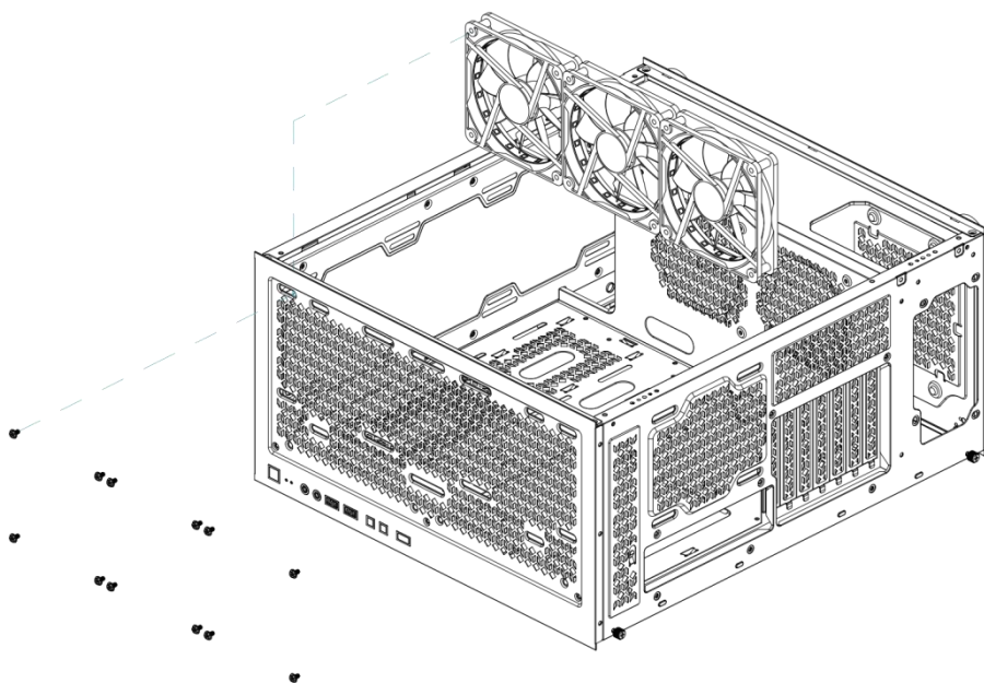
Installing the top fan
