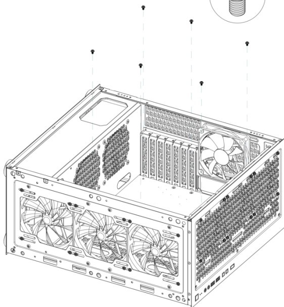
Instalacja płyty głównej
