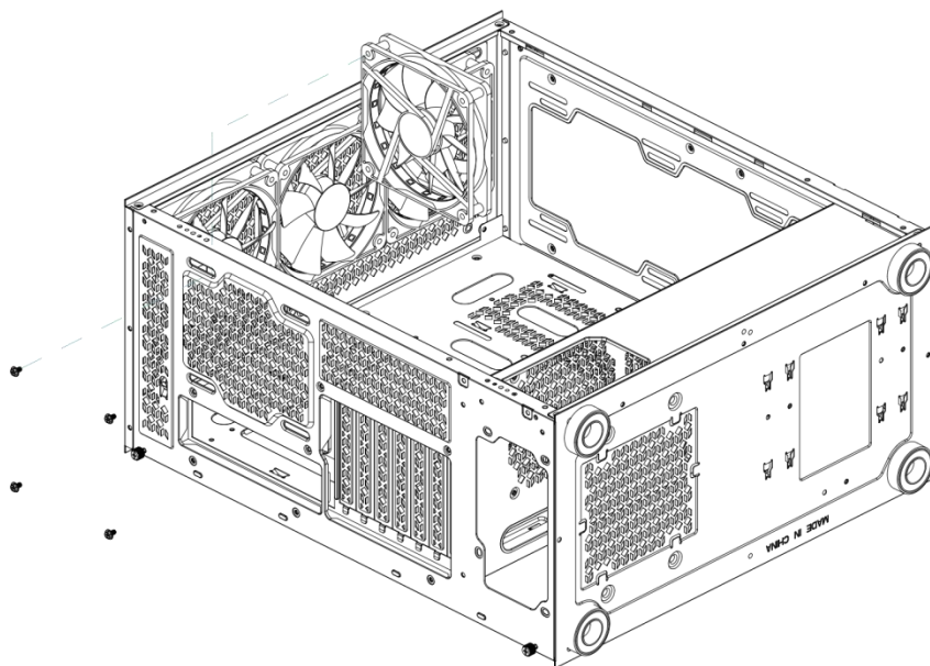
Installieren des hinteren Lüfters
