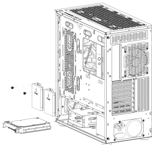
Instalowanie dysków twardych SSD i HDD
