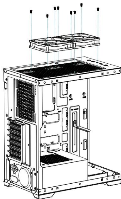
Installazione della ventola superiore
