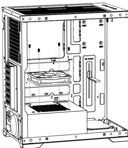
Installieren des oberen Lüfters des Netzteilfachs
