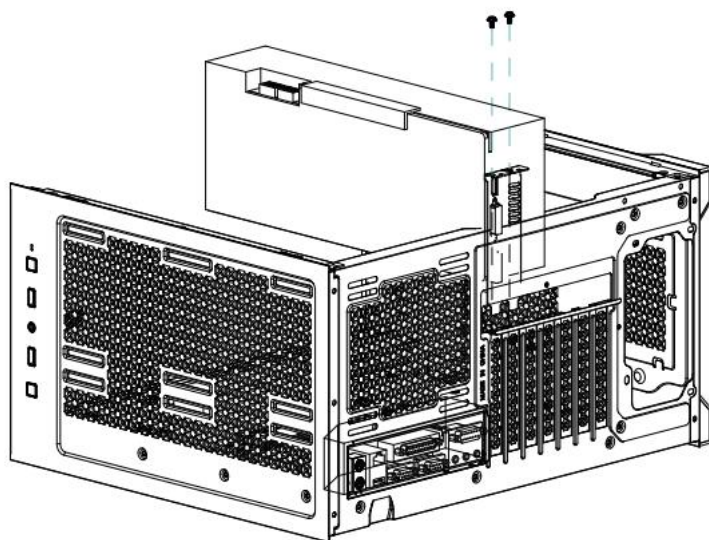
Installieren einer Grafikkarte
