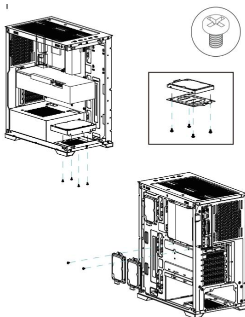
Installation de disques durs SSD et HDD
