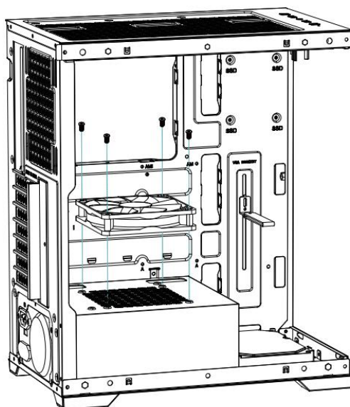
Instalación del ventilador superior del compartimento de la fuente de
