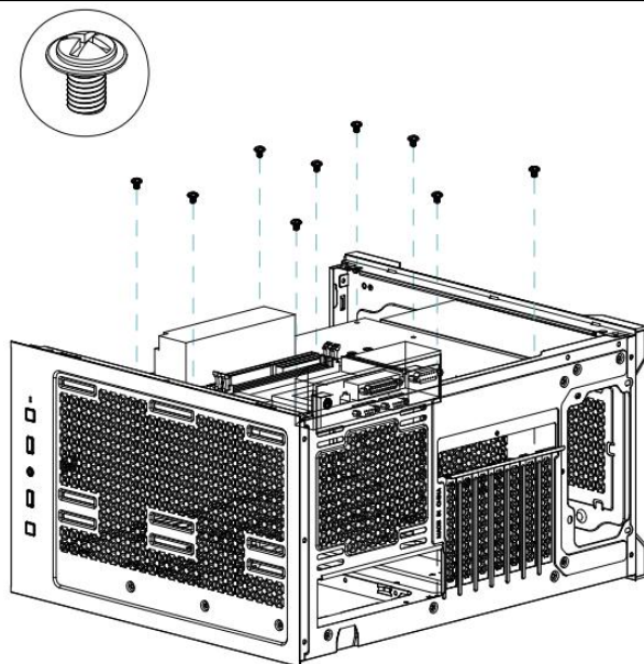
Installation de la carte mère
