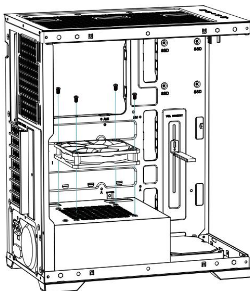
Installazione della ventola superiore del vano alimentatore
