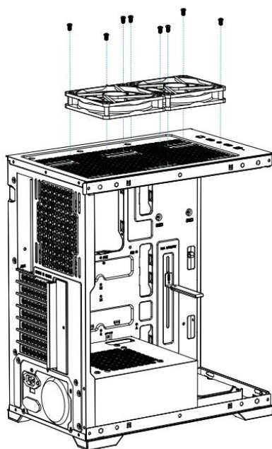
Installing the top fan
