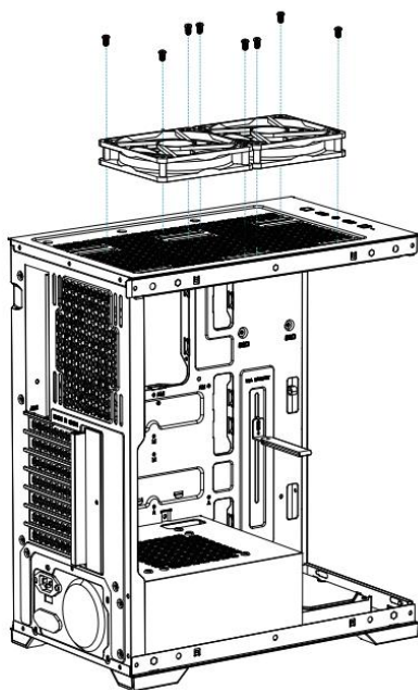
Installation av den övre fläkten
