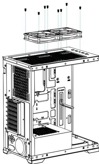
Instalación del ventilador superior
