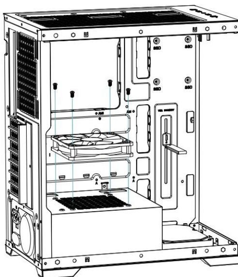
De bovenste ventilator van het voedingscompartiment installeren
