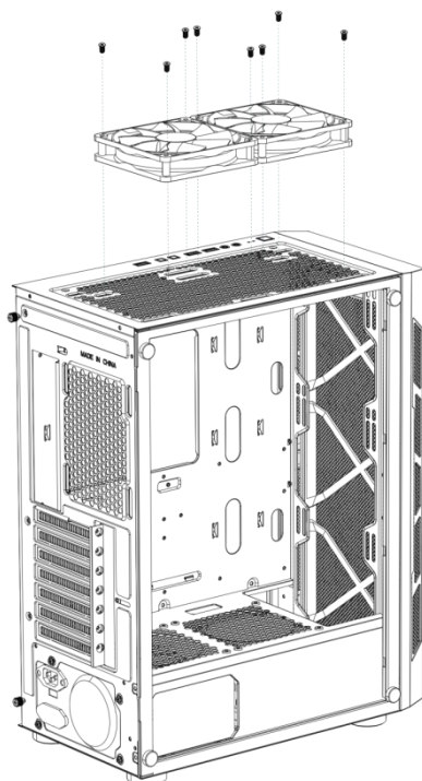
Installation du ventilateur supérieur
