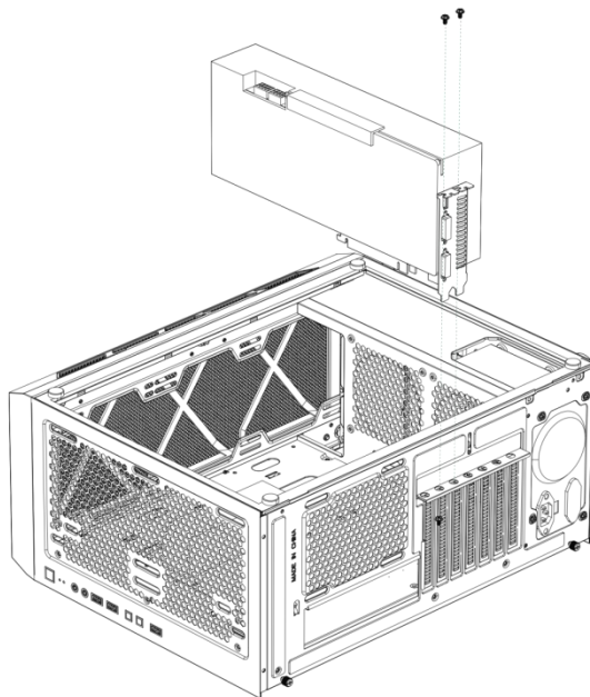
Instalowanie karty graficznej
