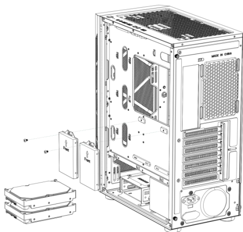
Installation av SSD- och HDD-hårddiskar
