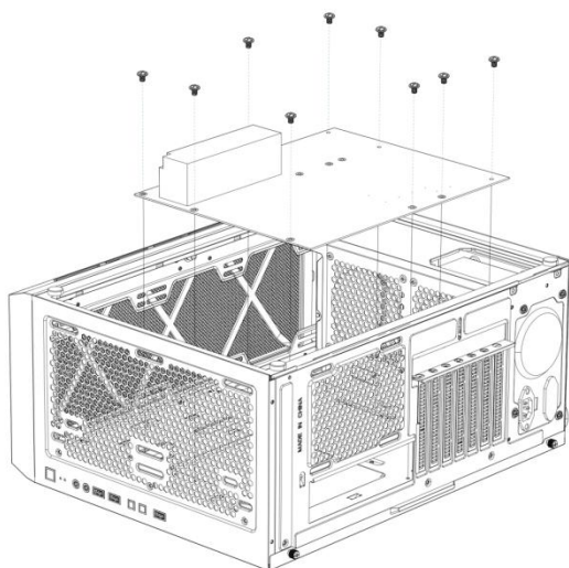
Installation av moderkortet
