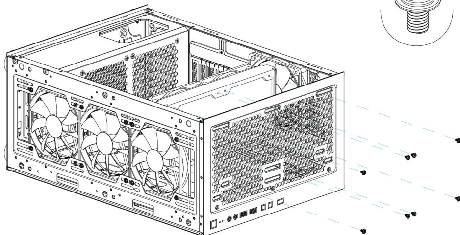
Installation av främre/bakre panelfläkten
