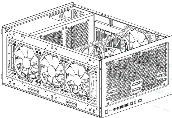
Installieren des oberen Lüfters
