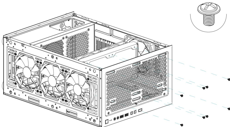
Instalación del ventilador del panel frontal/trasero
