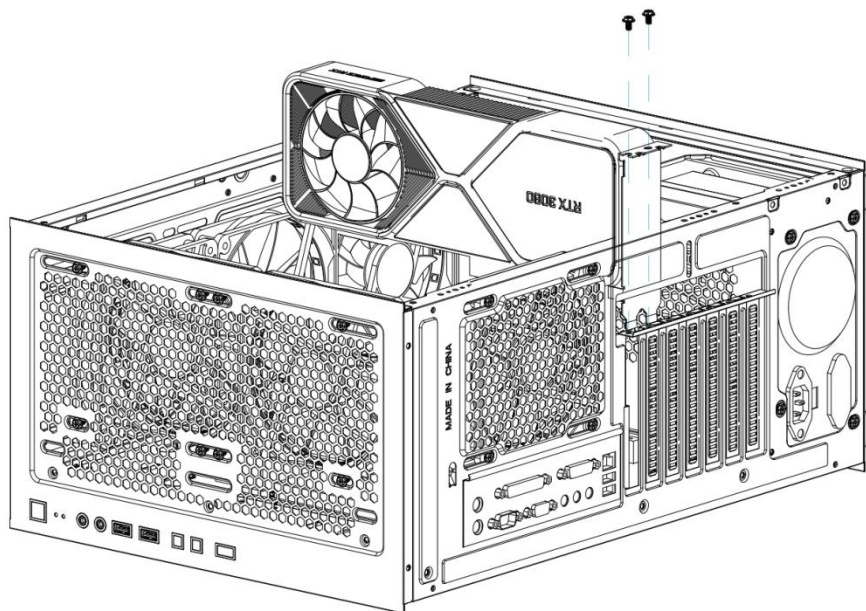
Instalowanie karty graficznej
