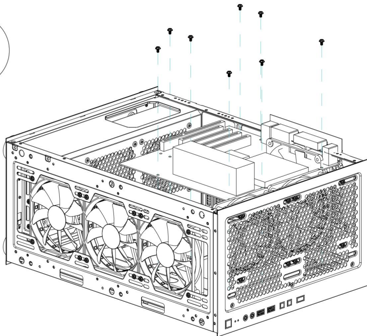
Installieren des Motherboards
