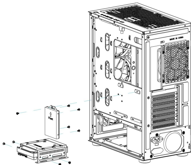
Installieren von SSD- und HDD-Festplatten
