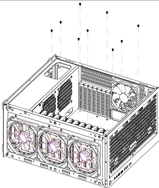
Installation de la carte mère
