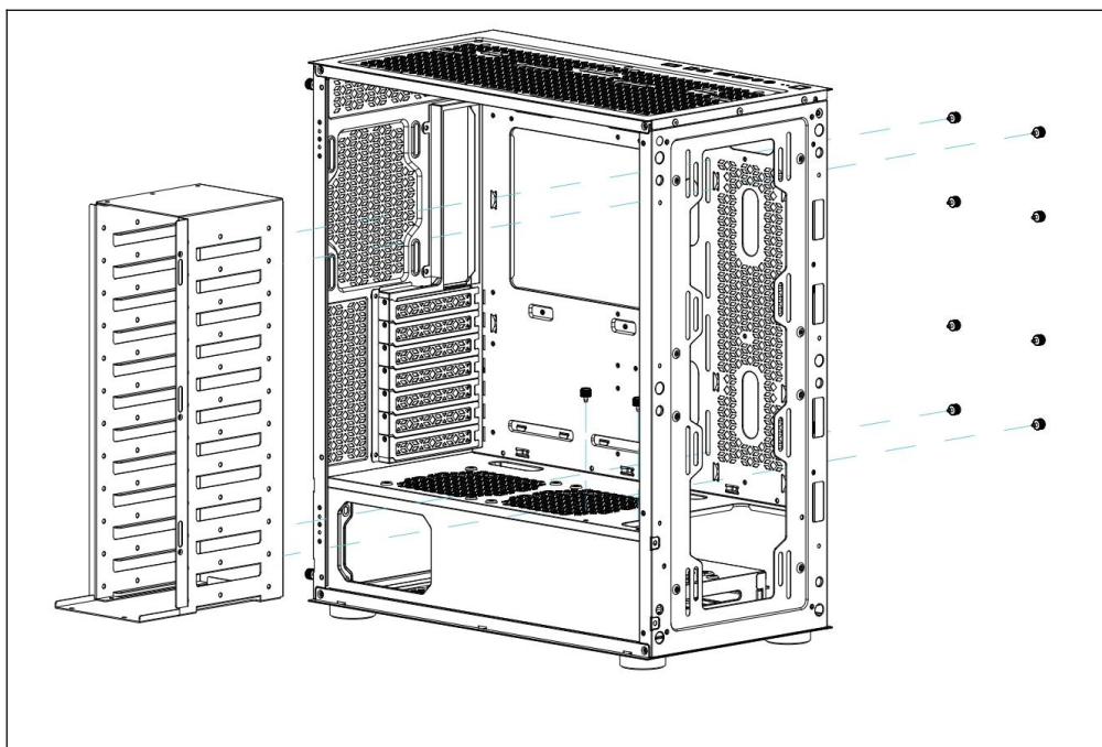
Smontaggio del rack del disco rigido
