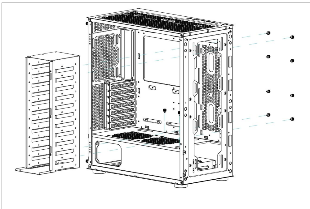
Démontage du rack de disque dur
