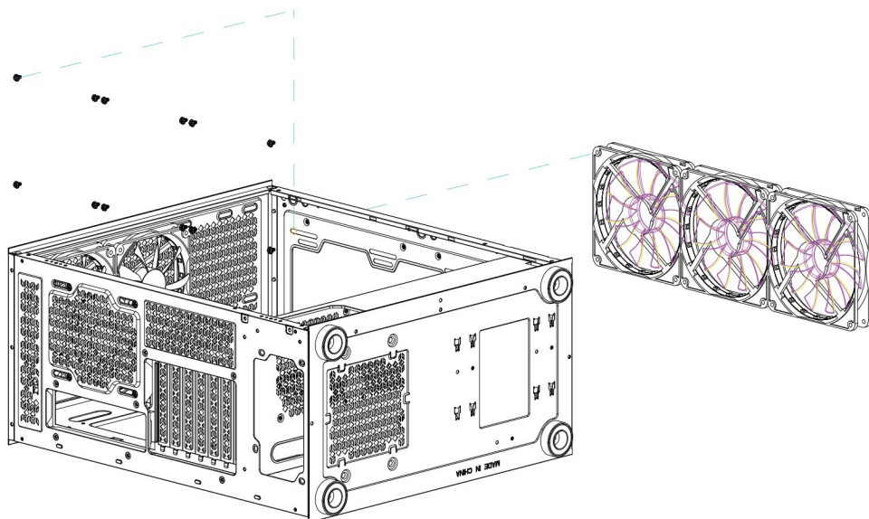
De achterste ventilator installeren
