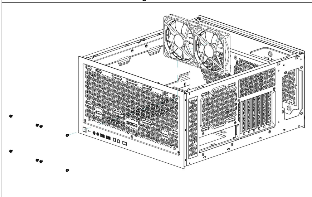
Installation av den övre fläkten
