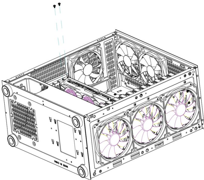
Een grafische kaart installeren
