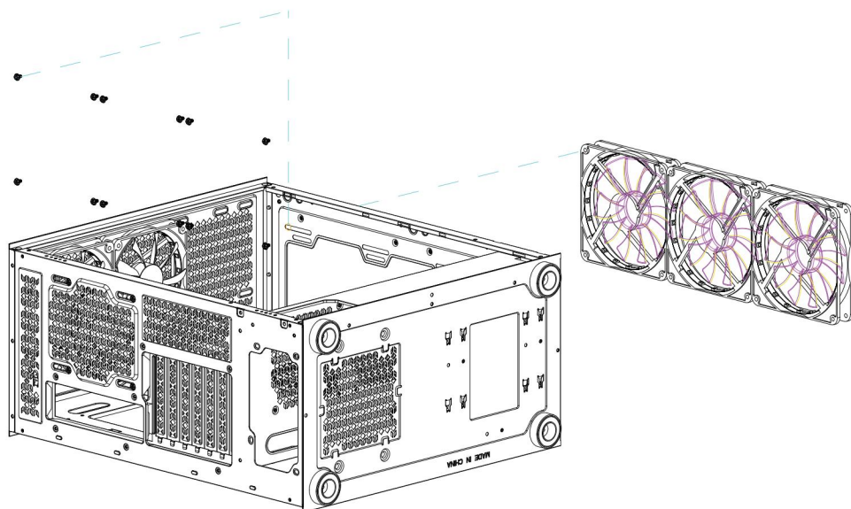
Montaż tylnego wentylatora
