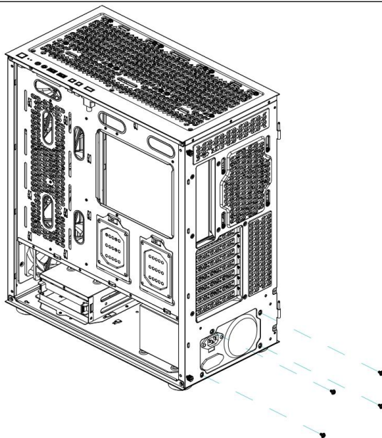
Instalación de la fuente de alimentación
