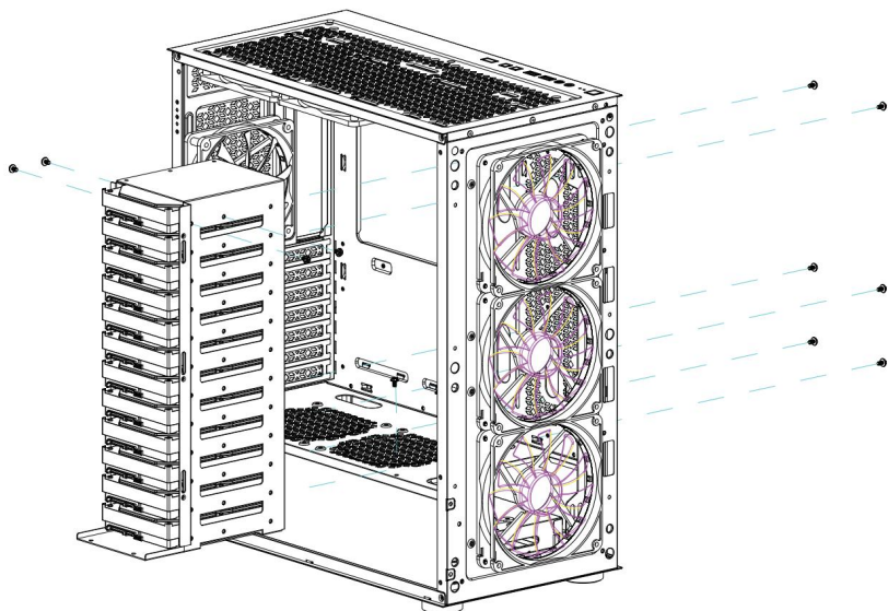
Instalación de discos duros
