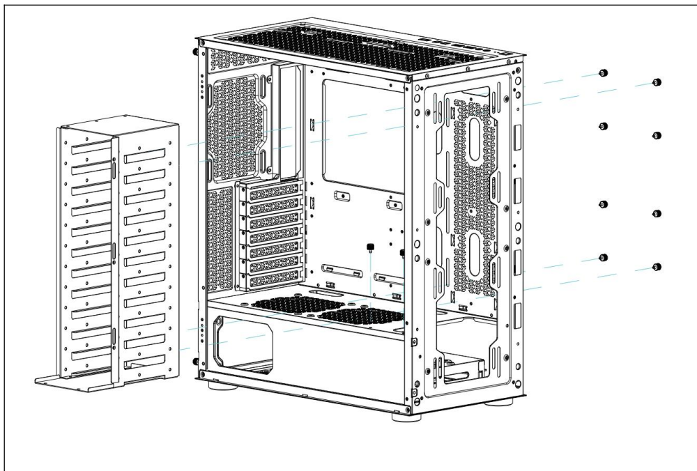
Demontage van het harde schijftek
