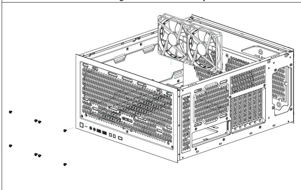
De bovenste ventilator installeren
