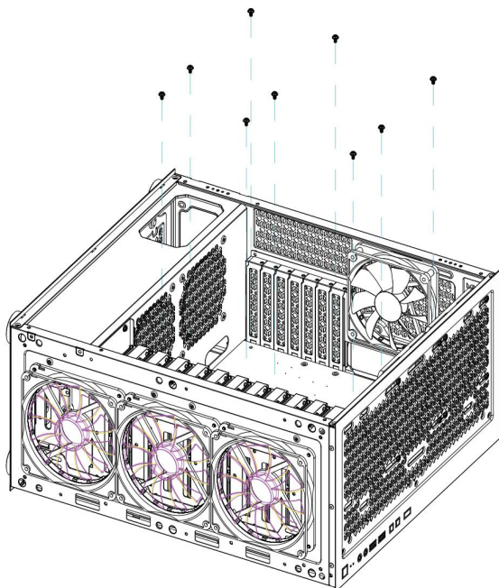
Installation av moderkortet
