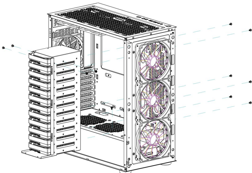
Installieren von Festplatten
