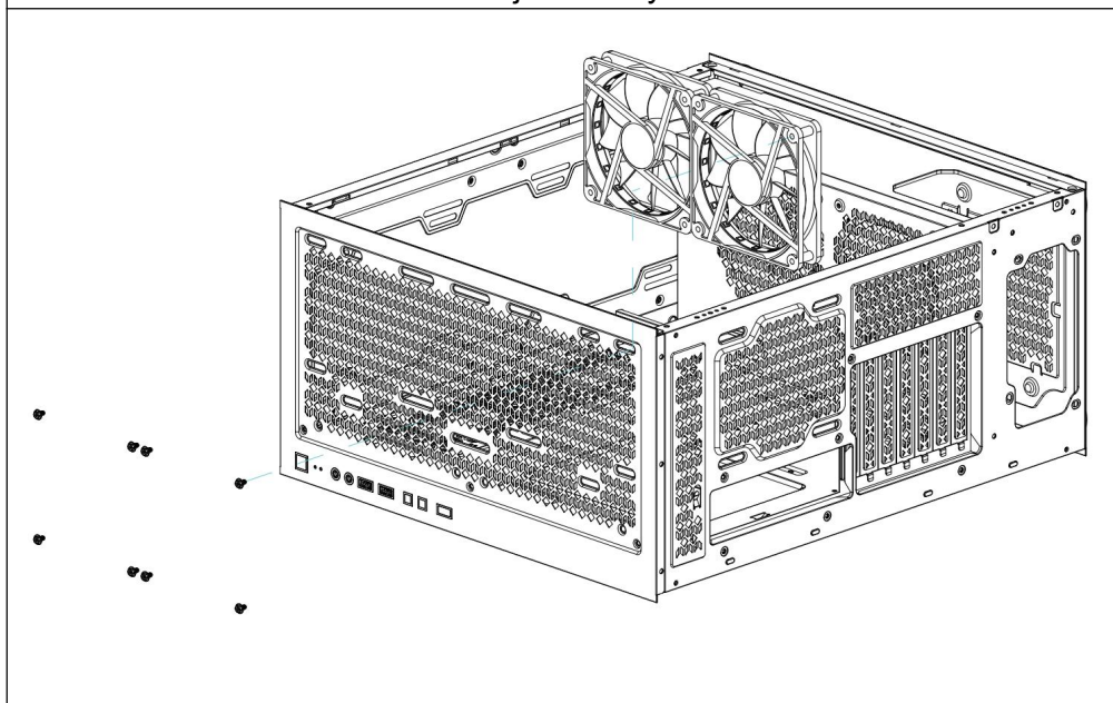
Montaż górnego wentylatora
