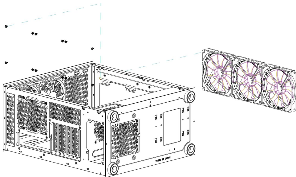
Installazione della ventola posteriore
