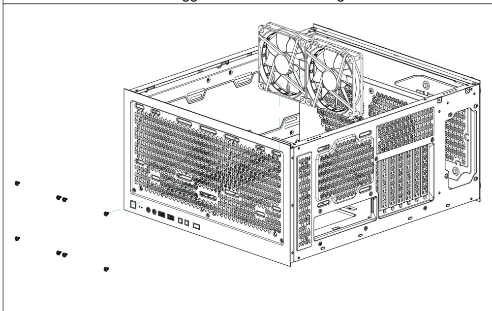
Installazione della ventola superiore
