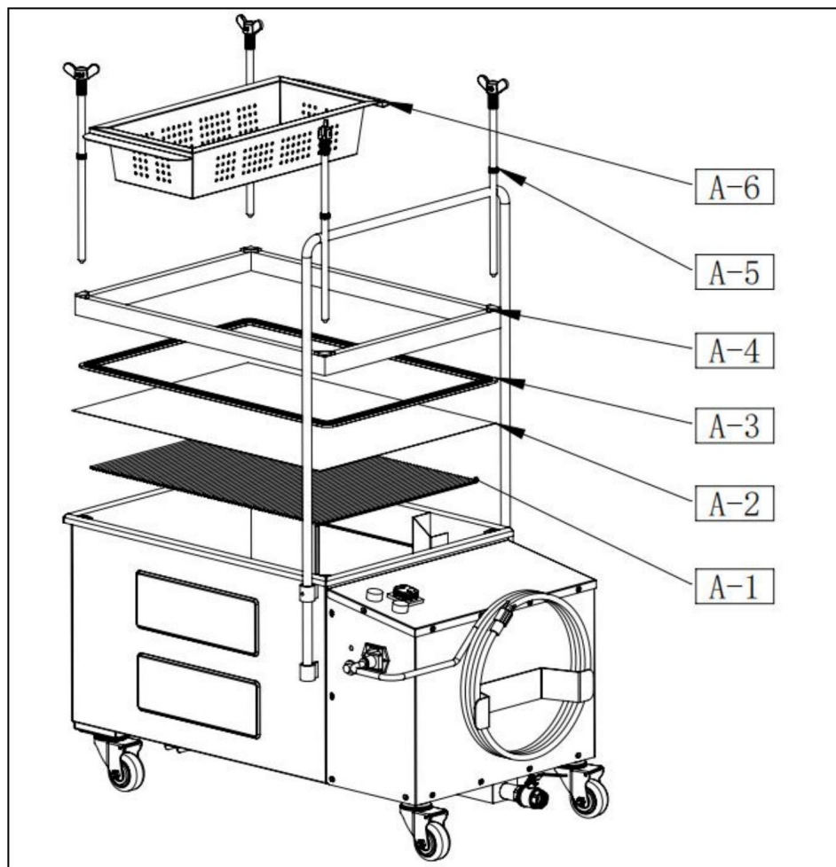
A-1:Filter A-2: Filterpapier A-3: Silikonkissen A-4: Drucksiebrahmen A-5: Filterkammerverstärkung A-6:Primärfilter
