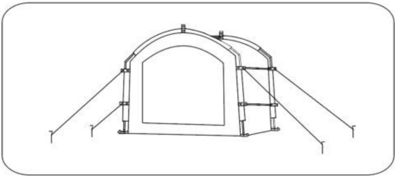
FASE 5: Chiodo di messa a terra della fune antivento fissa
