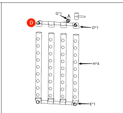
Figure 2 : Connectez un ensemble de tubes composites de connecteur , quatre canalisations de plantation, un ensemble
