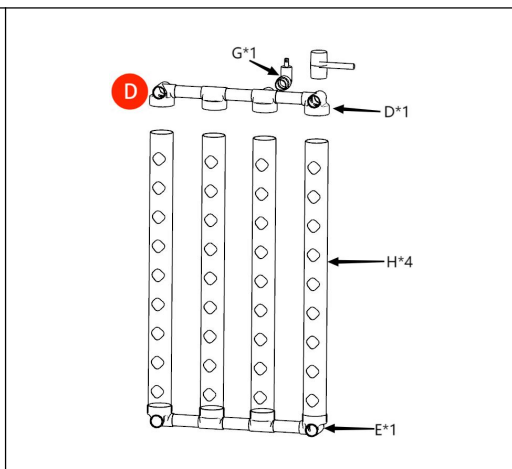
Figur 2: Anslut en uppsättning kompositrör för kopplingar , fyra planteringsrörledningar, en uppsättning kompositrör för vattenutlopp med bokstaven D och en utloppskran enligt diagrammet, med planteringsrörledningarna vända uppåt. Förstärk dem med en gummihammare
