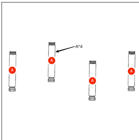
Figura 1: Prepare cuatro tubos de pie de 300 mm.
