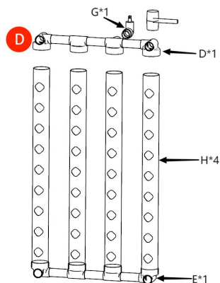
Figuur 2: Sluit een set samengestelde verbodingsbuizen , vier plantpijpleidingen, een set samengestelde waterafvoerpijpen met de letter D en een uitlaatkraan aan elkaar volgens het diagram, met de
