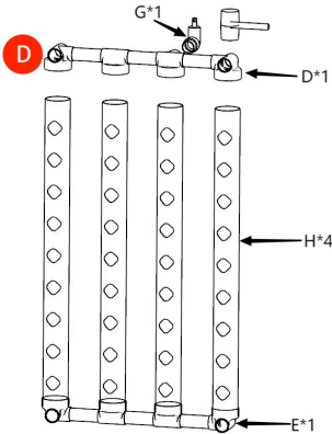
Figura 2: Collegare insieme un set di tubi composti di collegamento , quattro tubazioni per la semina, un set di tubi
