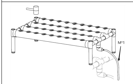
Figura 3: Conecte el conjunto de la Figura 2 y los cuatro tubos de pie de la Figura 1 juntos, y conecte una manguera de salida de agua de 1 m al grifo de salida. La manguera debe
