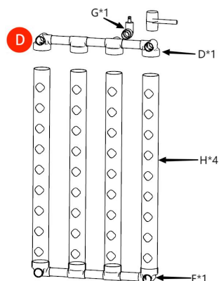
Abbildung 2: Verbinden Sie einen Satz Verbindungs-Verbundrohre , vier Pflanzrohre, einen Satz Wasserauslass-Verbundrohre mit dem Buchstaben D und einen Auslasshahn gemäß der Abbildung miteinander, wobei
