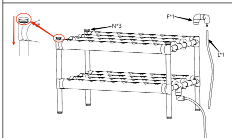
Figure 7 : Connectez ensemble trois bouchons anti-poussière, un robinet d'arrivée et un tuyau de 1,5 m selon le schéma. Le tuyau doit être coupé à la longueur appropriée et maintenu droit pour éviter d'affecter le débit.
