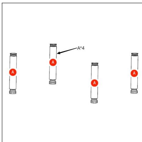
Abbildung 1: Bereiten Sie vier 300-mm-Fußrohre vor.
