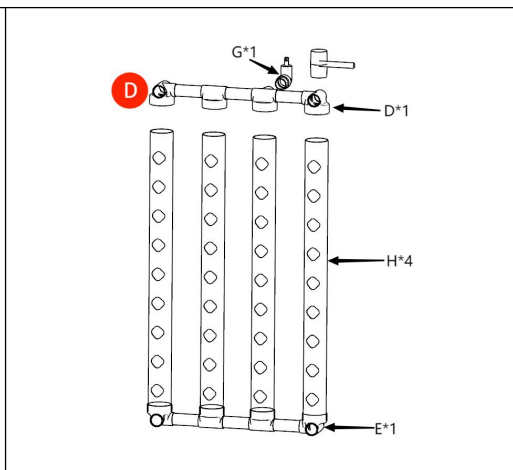
Figura 2: Conecte un conjunto de tubos compuestos conectores , cuatro tuberías de plantación, un conjunto de tuberías compuestas de salida de agua con la letra D y un grifo de salida según el diagrama, con las tuberías de plantación hacia arriba. Refuézalos con un martillo de goma (golpea cada conexión con el martillo de goma hasta que encajen bien)
