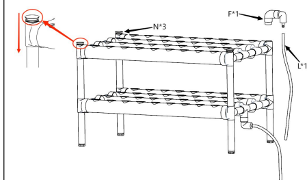
Figura 7: Collegare insieme tre tappi antipolvere, un rubinetto di ingresso e un tubo flessibile da 1,5 m secondo lo schema. Il tubo deve essere tagliato alla lunghezza adeguata e mantenuto dritto per evitare di influenzare la portata.
