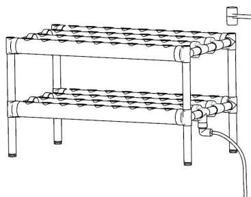
Figura 6: Collegare insieme il gruppo della Figura 5 e il gruppo della Figura 4. (Rinforzare i quattro angoli con un martello di gomma per regolare il livello)
