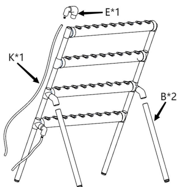
Figur 3: Anslut två 520 mm fotrör, en 1,5 m slang och en inloppskran med enheten i figur 2 enligt diagrammet.
