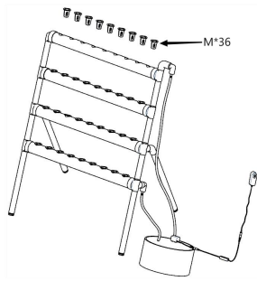
Bild 6: Sätt 36 planteringskorgar i planteringsrörledningarna och sätt in adaptorn i strömförsörjningen. När vattenpumpen fungerar kommer den att bilda en vattenflödescykel. Justera slutligen balansen på fötterna så att det rinner
