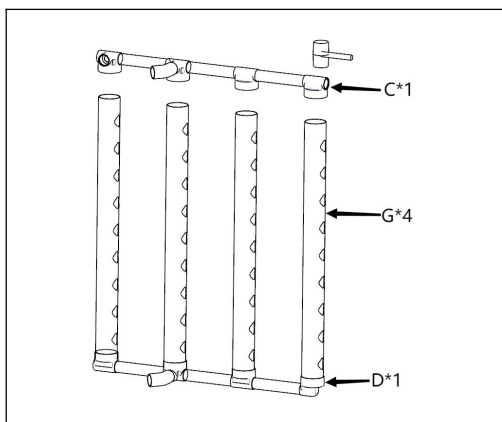
Figur 1: Anslut en uppsättning kompositrör för kopplingar , en uppsättning kompositrör för vattenutlopp och fyra planteringsrörledningar tillsammans enligt diagrammet, med
