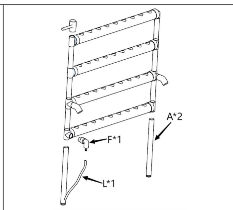
Figur 2: Anslut två 400 mm fotrör, en 1 m slang och en utloppskran med enheten i figur 1 enligt diagrammet. (Förstärk de två vinklarna med en gummihammare för att justera nivån)
