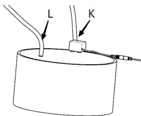
Bild 5: Förbered först en vattentank och fyll den med vatten. (Det rekommenderas att använda en vattentank som har en kapacitet på mer än 20L, vilket inte inkluderar 20L). Anslut den andra änden av 1,5 m slangen till vattenpumpen och fäst
